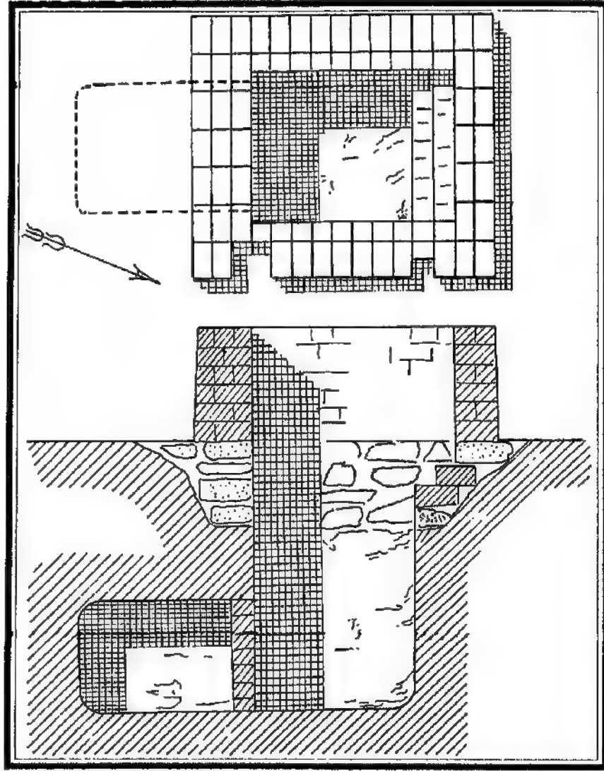
(شكل ٩٧) مسقطان أفقى ورأسى لبقبرة الطبقة الفقيرة فى أواخر الأسرة الثانية.
